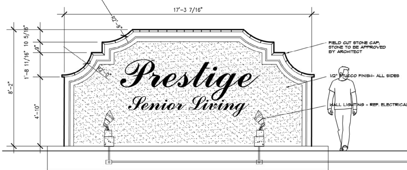
4 A1.1 SCALE: 1/4" = 1'-0"
