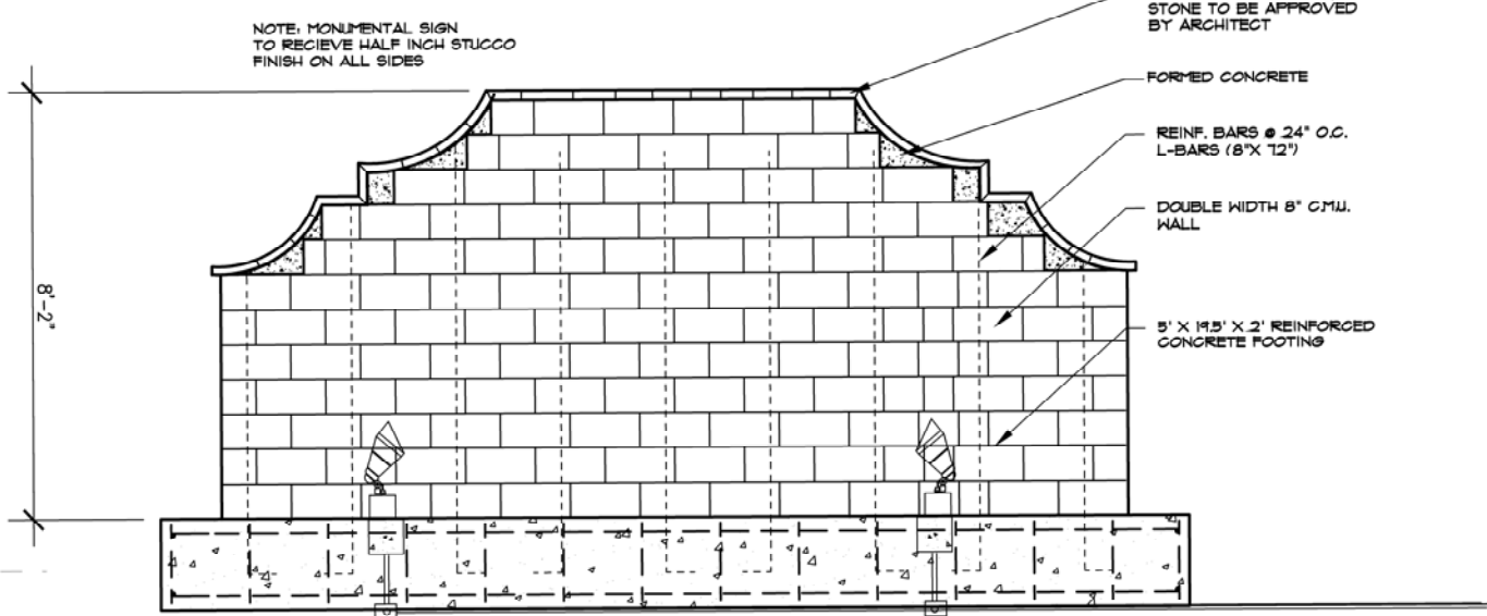
5 A1.1 SCALE: 1/4" = 1'-0"
