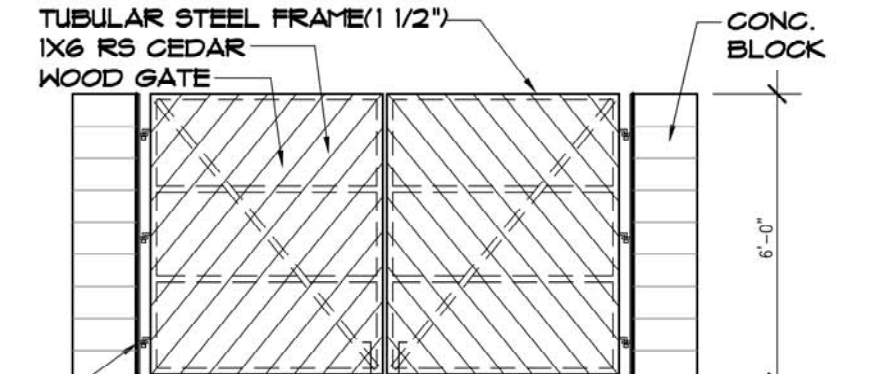
BACK ELEVATION SCALE: 1/4"=1'-0"
