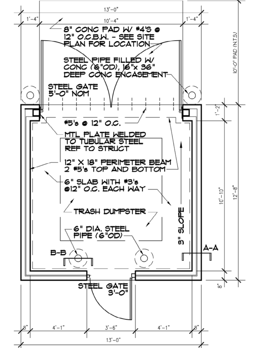
PLAN SCALE: 1/4"=1'-0"
