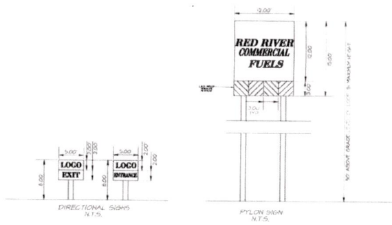
SIGN ELEVATIONS N.T.S.
